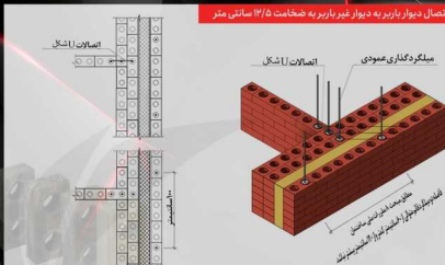
نحوه اتصال دیوار باربر به دیوار غیر باربر به ضخامت ۱۲/۵ سانتی متر
