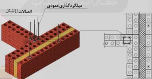
نحوه اتصال دو دیوار باربر به یکدیگر
