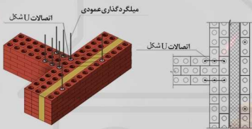
نحوه اتصال دو دیوار باربر به یکدیگر
